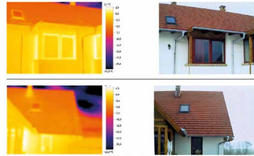
▲ Hőkamerás felvétel, préselt földtégla lakóházról. Az értékek megfelelőek.
